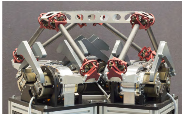
(d) University of Twente - Netherlands [99]
