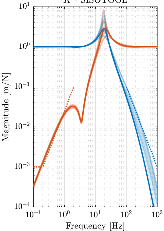
K - SISOTOOL
